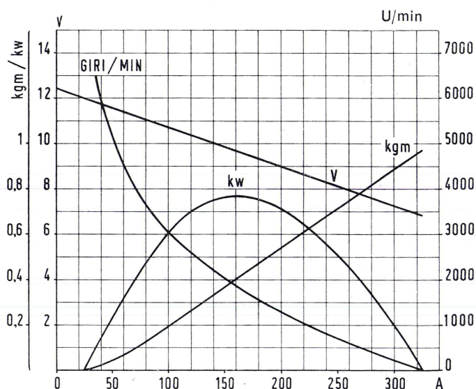
Abb. 74. - Leistungskurven des Anlassers FIAT E 100-1,3/12.
