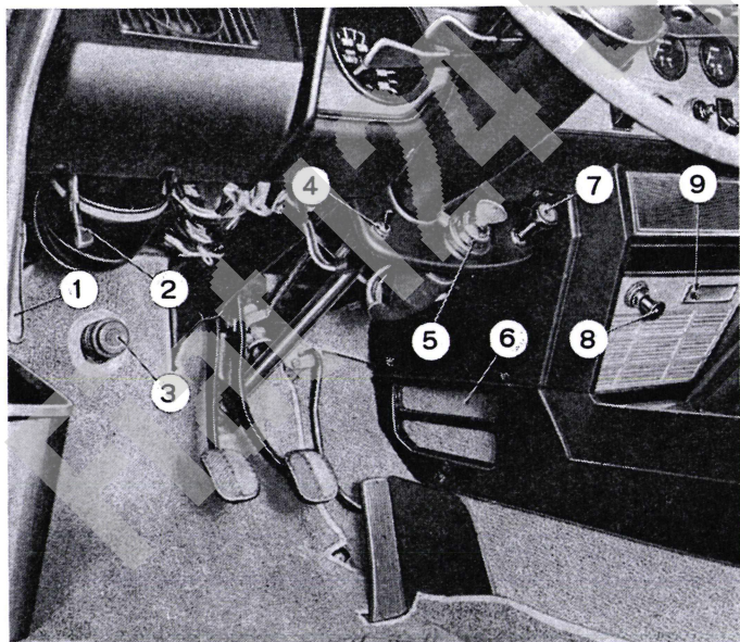
Abb. 103. - Teilansicht auf die Betätigungsorgane.
