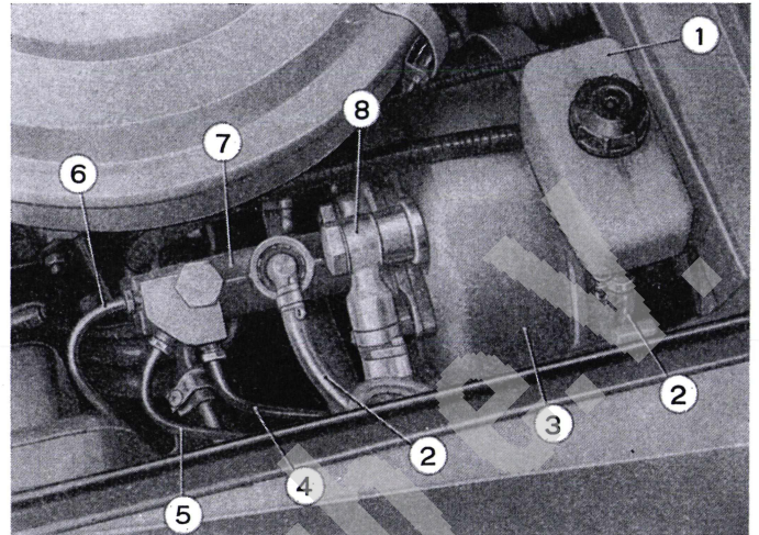
Abb. 57. - Anordnung der Master-Vac-Servobremse im Wagen
