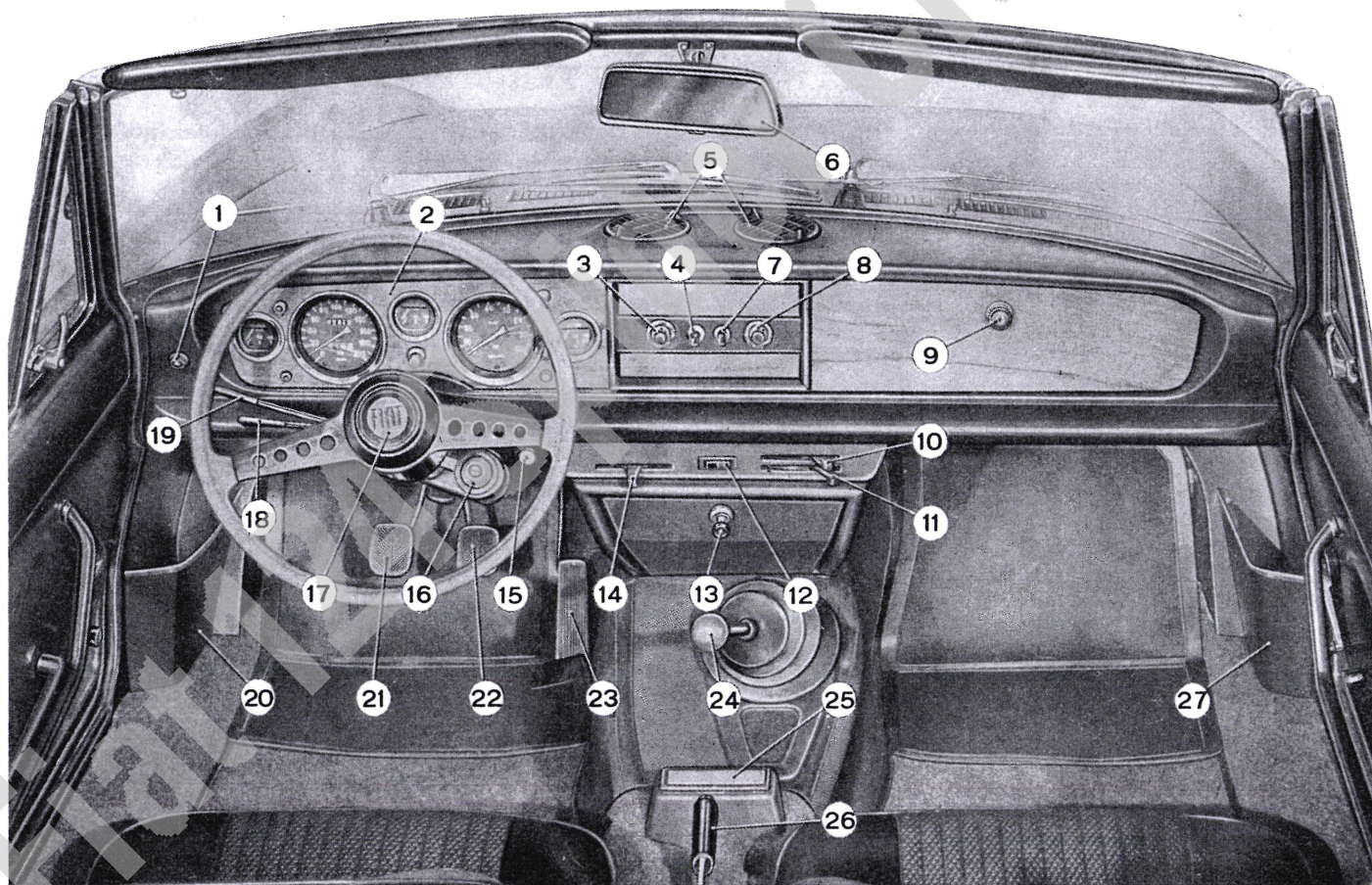
Abb. 64. - Anordnung der Kontroll-, Signal- und Betätigungsorgane.
