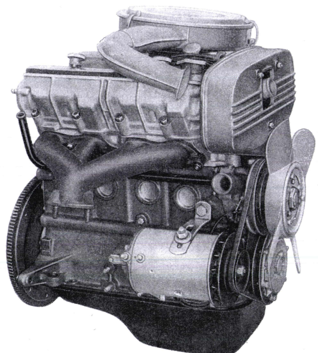
Abb. 4. - Vordere rechte Seite des Motors.
