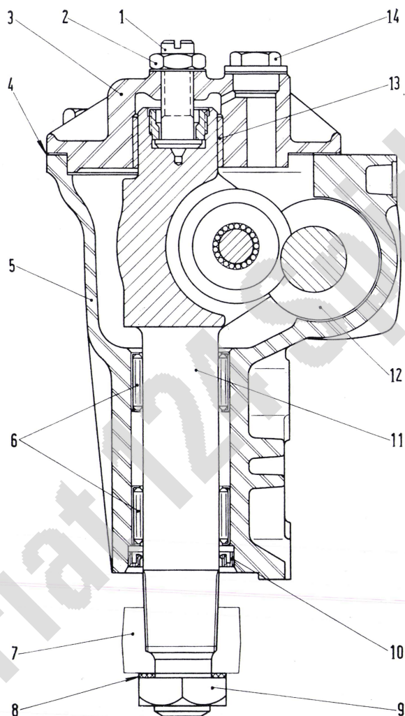
Abb. 95. - Schnitt des Lenkgetriebes, Ersatzteilbestellnummer 4167806, durch die Lenkrollenwelle.
