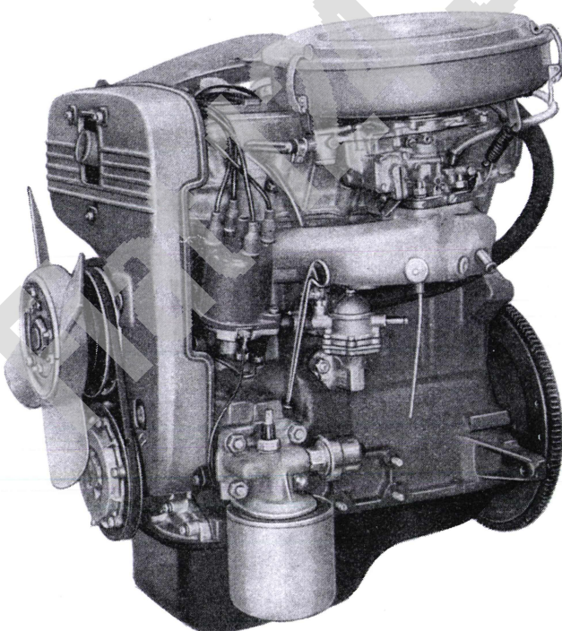
Abb. 3. - Vordere linke Seite des Motors.
