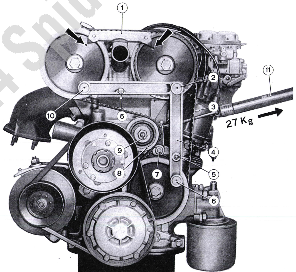
Abb. 29. - Montage und Einstellung des gezahnten Treibriemens zum Antrieb der Nockenwellen und der Antriebswelle für die Hilfsorgane.
