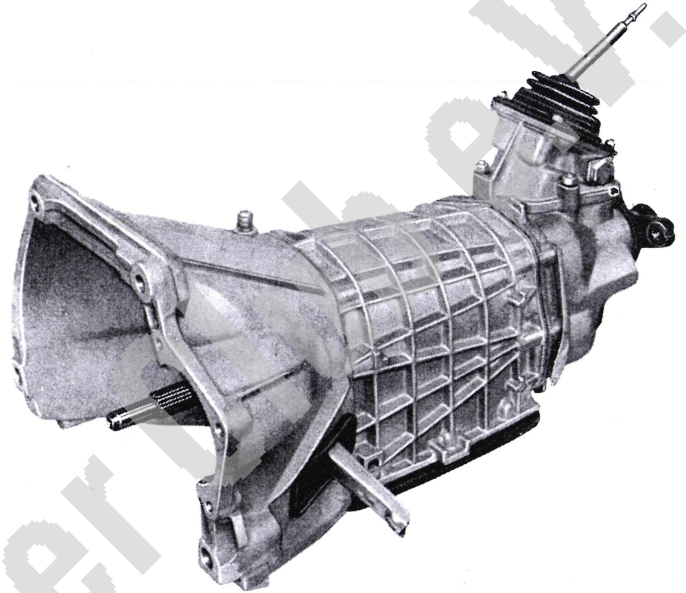
Abb. 40. - Gesamtansicht des Wechselgetriebes.
