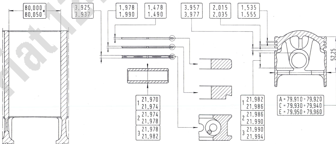
Abb. 6. - Hauptdaten der Zylinder, des Pleuellagers, des Pleuellagerbolzens und des Pleuellagerbolzenmutter.
