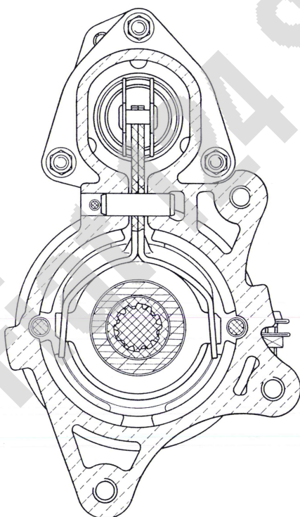
Abb. 80. - Querschnitt durch den Ritzeltrieb.
