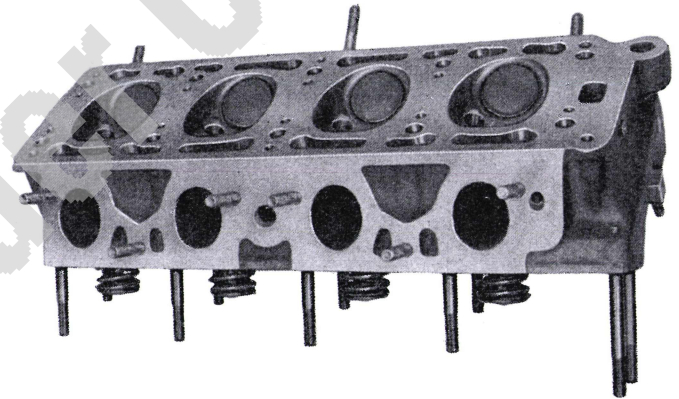
Abb. 16. - Ansicht des Zylinderkopfes von unten.
