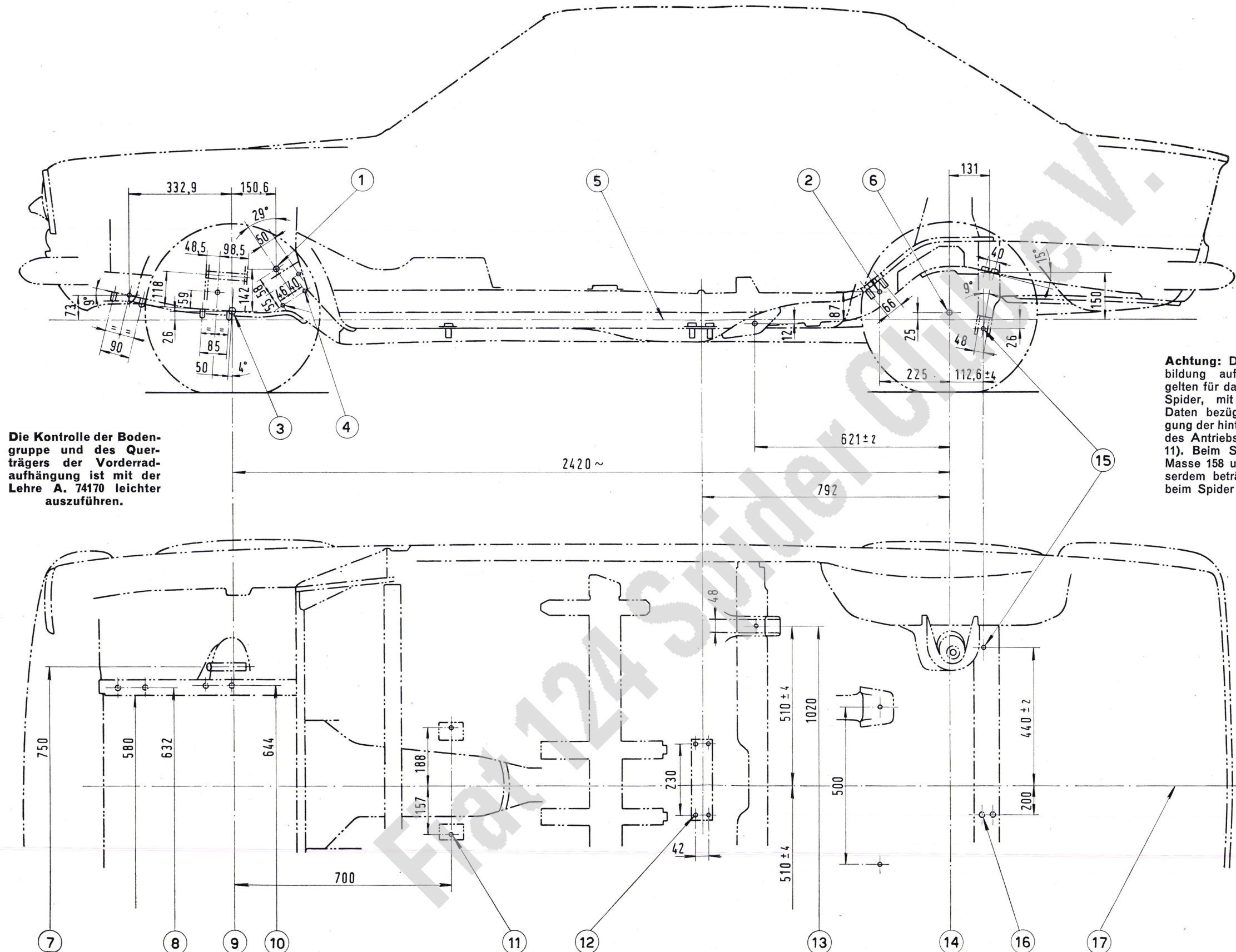
Abb. 99. - Hauptdaten zur Kontrolle der Befestigungspunkte der mechanischen Gruppen an die Bodengruppe.
