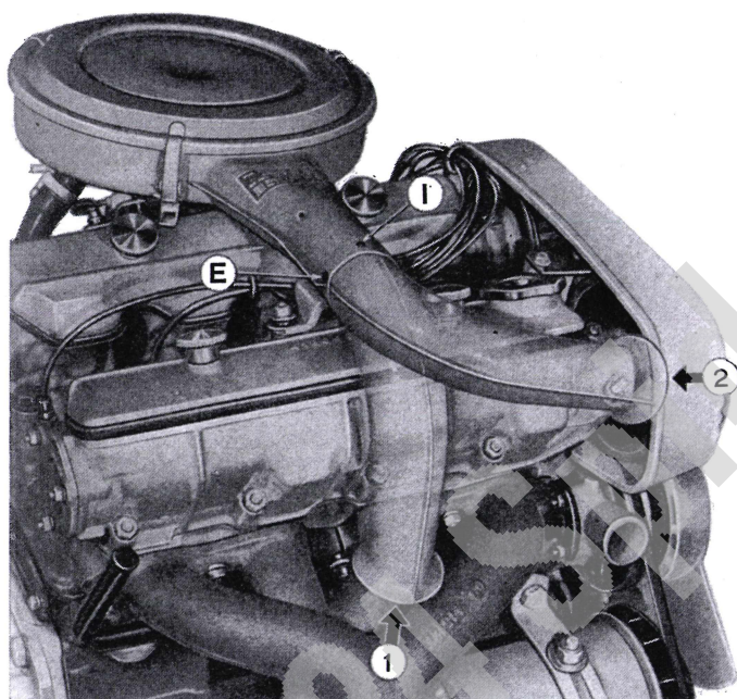
Abb. 33. - Jahreszeitliche Regelung der Luftzufuhr zum Luftfilter.
