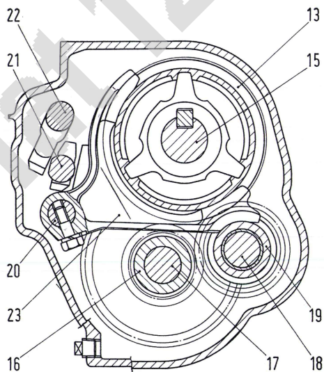
Abb. 46. - Querschnitt durch die Schaltung des fünften Ganges.
