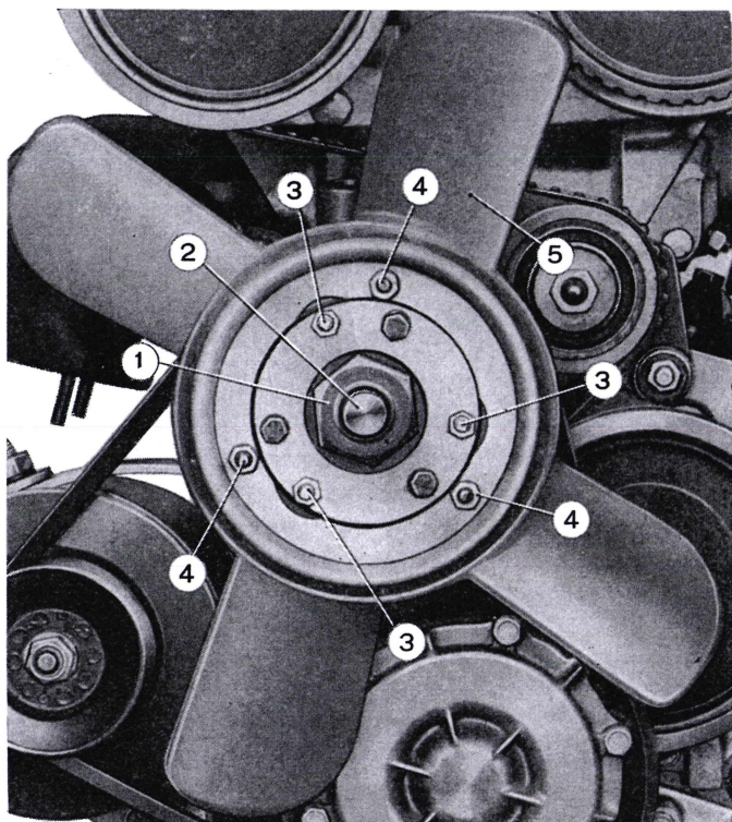
Abb. 37. - Elektromagnetisch ein- und ausgeschalteter Ventilator am Motor.
