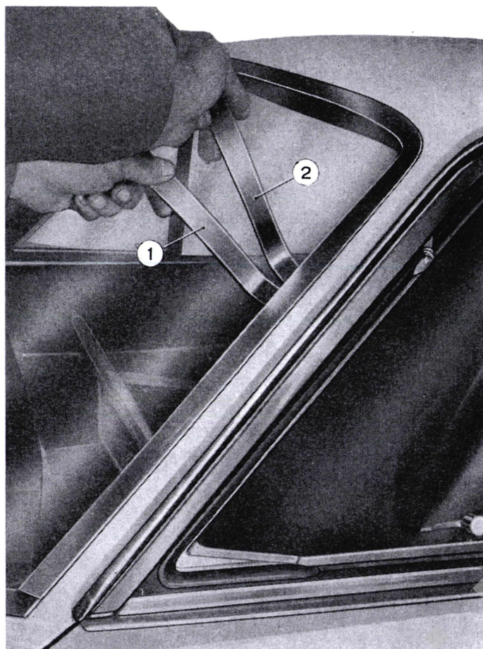
Abb. 114. - Anwendung der Werkzeuge A. 78032 zum Ausbau des Zierrahmens der Windschutzscheibe.
