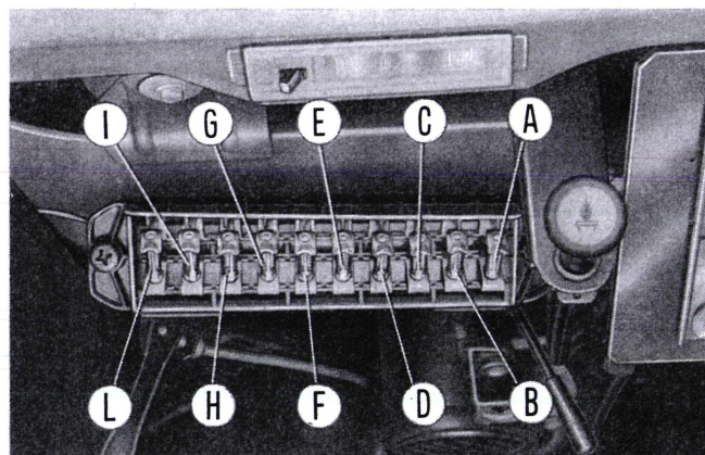
Abb. 90. - Schmelzsicherungen.
