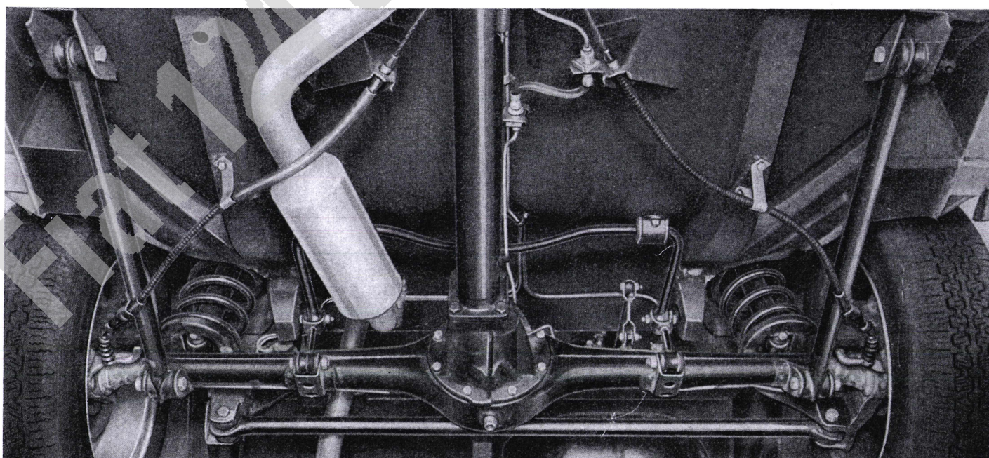
Abb. 55. - Hintere Aufhängung am Wagen montiert, von vorne gesehen.
