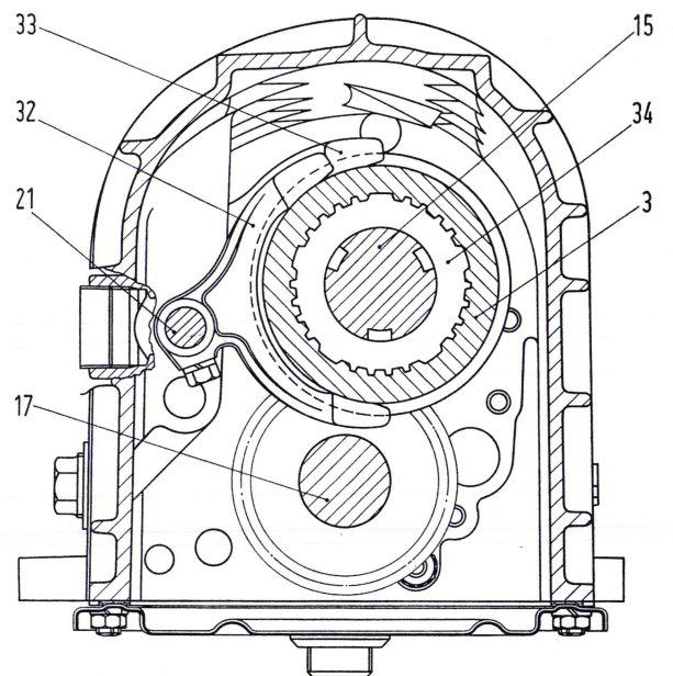
Abb. 48. - Querschnitt durch die Schiebemuffe für den 3. und 4. Gang.
