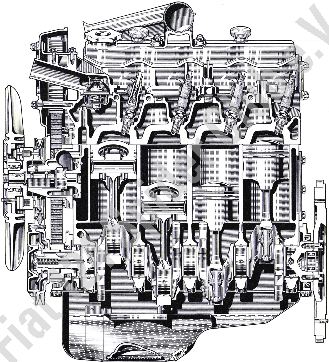
Abb. 7. - Längsschnitt durch die Zylinder des Motors.
