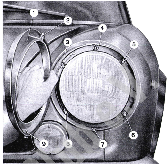
Abb. 106. - Linker Scheinwerfer.
