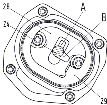
Abb. 44. - Schnitte durch das Lager für den Schalthebel.
